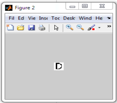
Fig.3. Input
